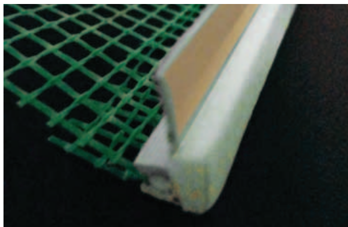
Kontakt lajsna sa staklenom mrežom
